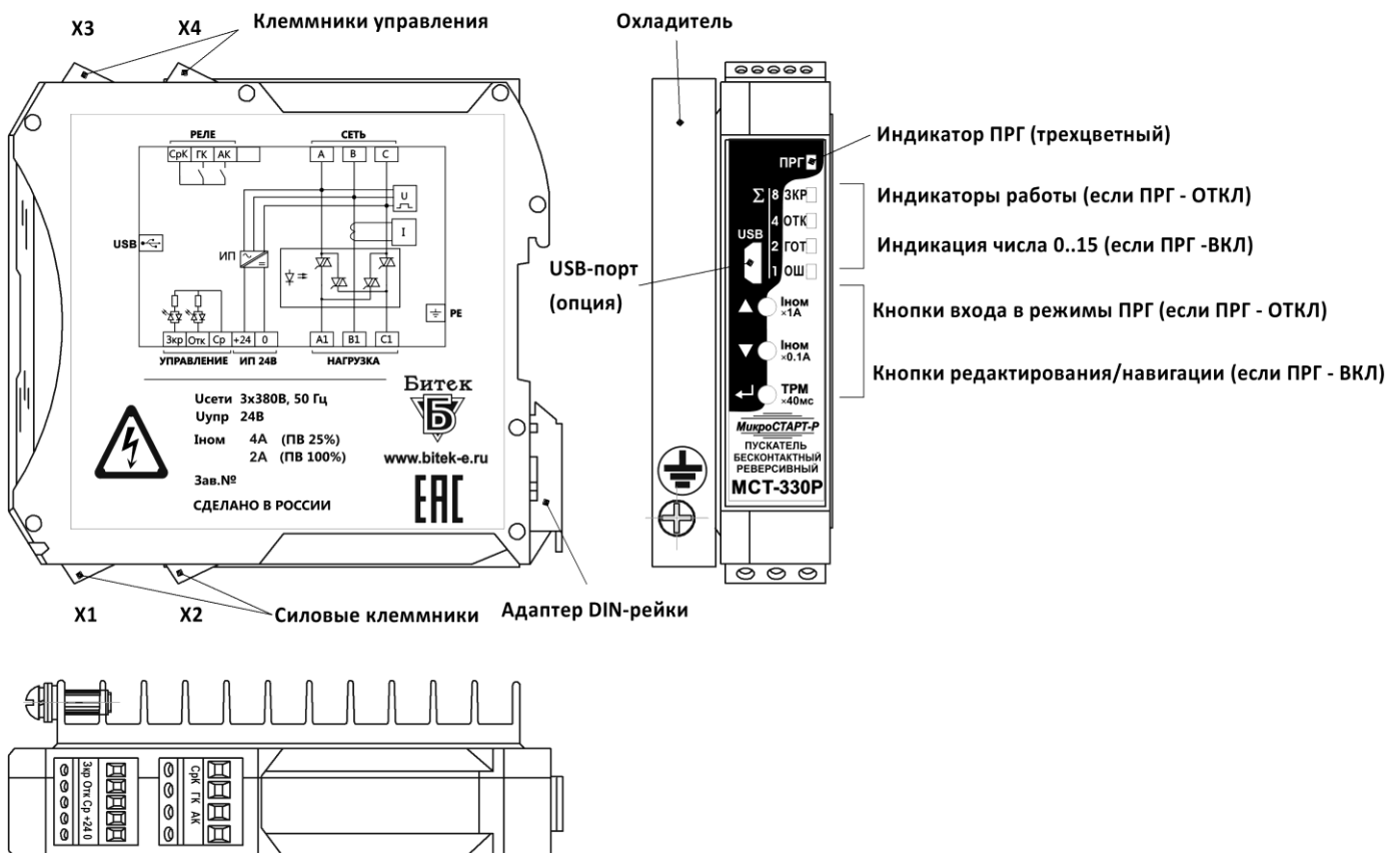
Рисунок 1 - Внешний вид пускателя МСТ-330P-USB
