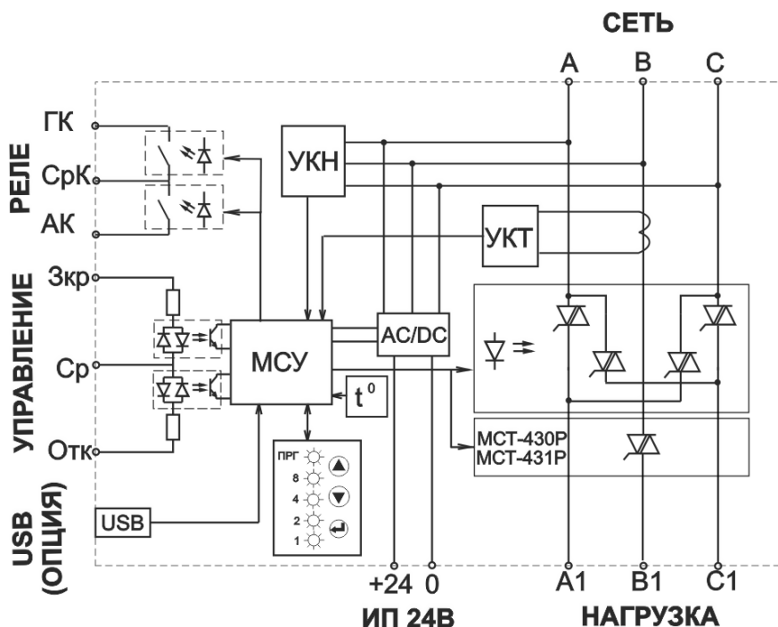
Рисунок 2 – Функциональная схема пускателей МСТ-330Р, МСТ-331Р, МСТ-430Р, МСТ-431Р
