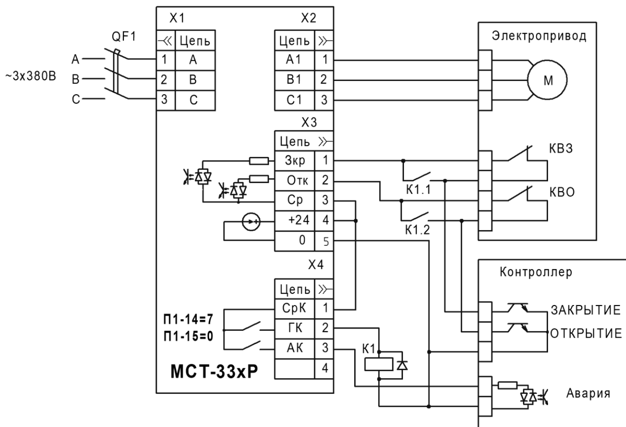
Рисунок 13 - Пример схемы подключения с функцией дожима задвижки
