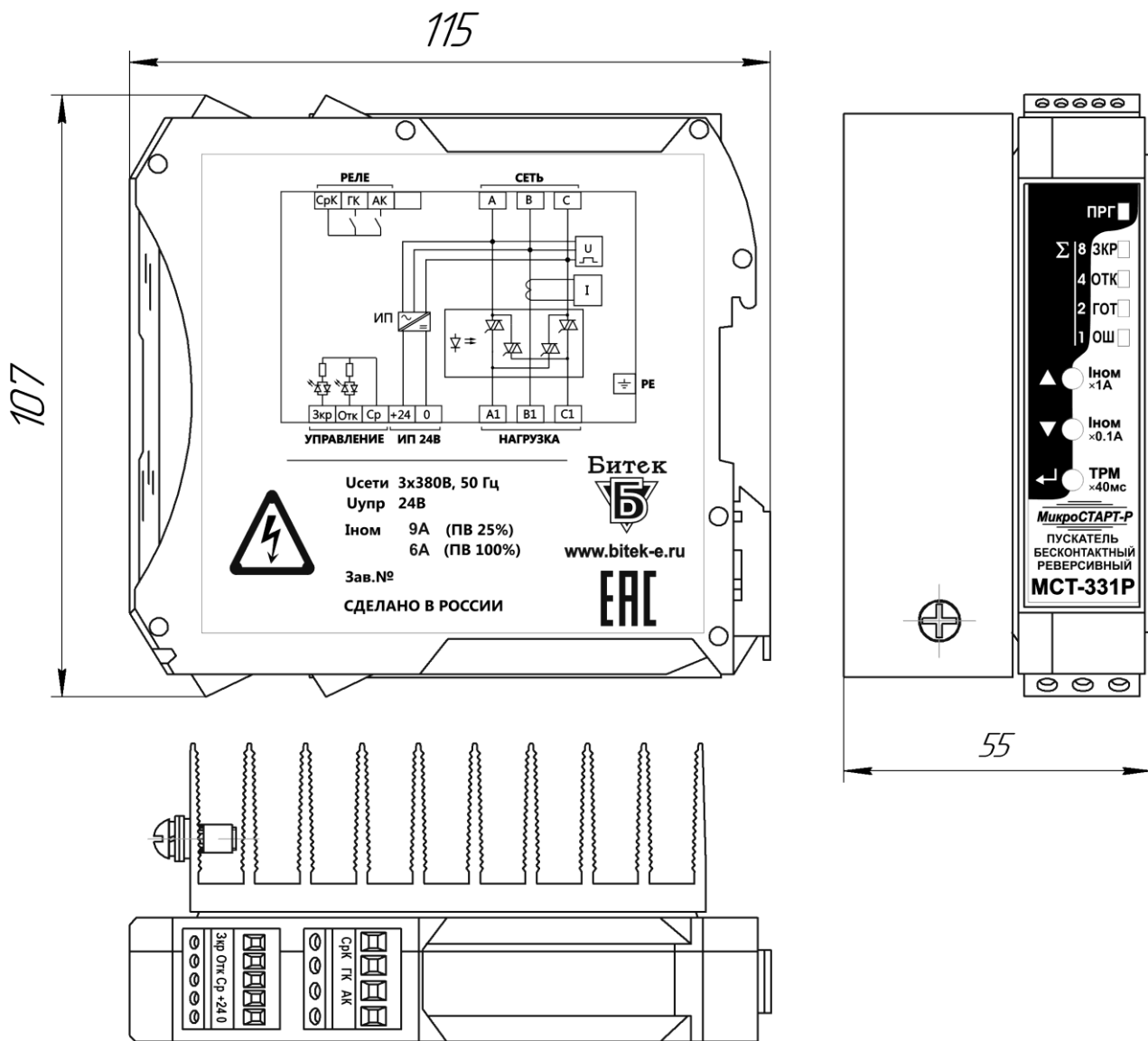
Рисунок А.2 – Габаритно-установочные размеры МСТ-331Р, МСТ-431Р
